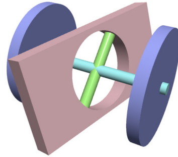
Fig. 3 車軸まわりの模式図．斜めに支持された十字の軸に車輪が取り付けられている．
