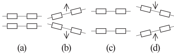
Fig. 2 移動の手順．足の方向を変えつつ，足の開閉を行う．
